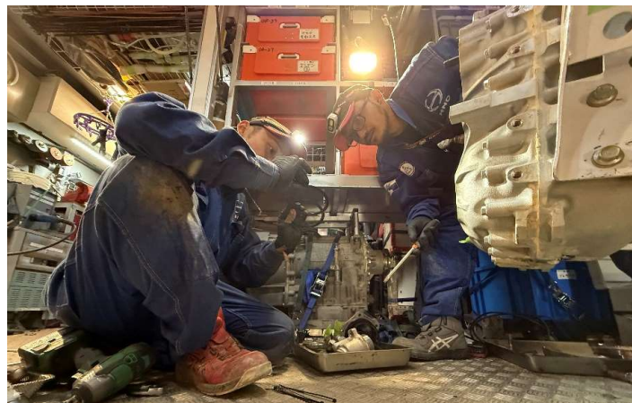
↑トランスファーの分解をする上原メカ(左)と柏谷メカ(右)
